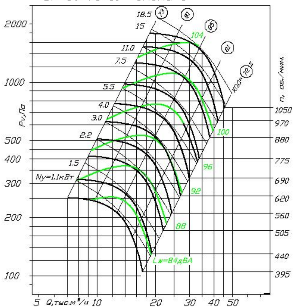
BP 80-75-10 схема 5
