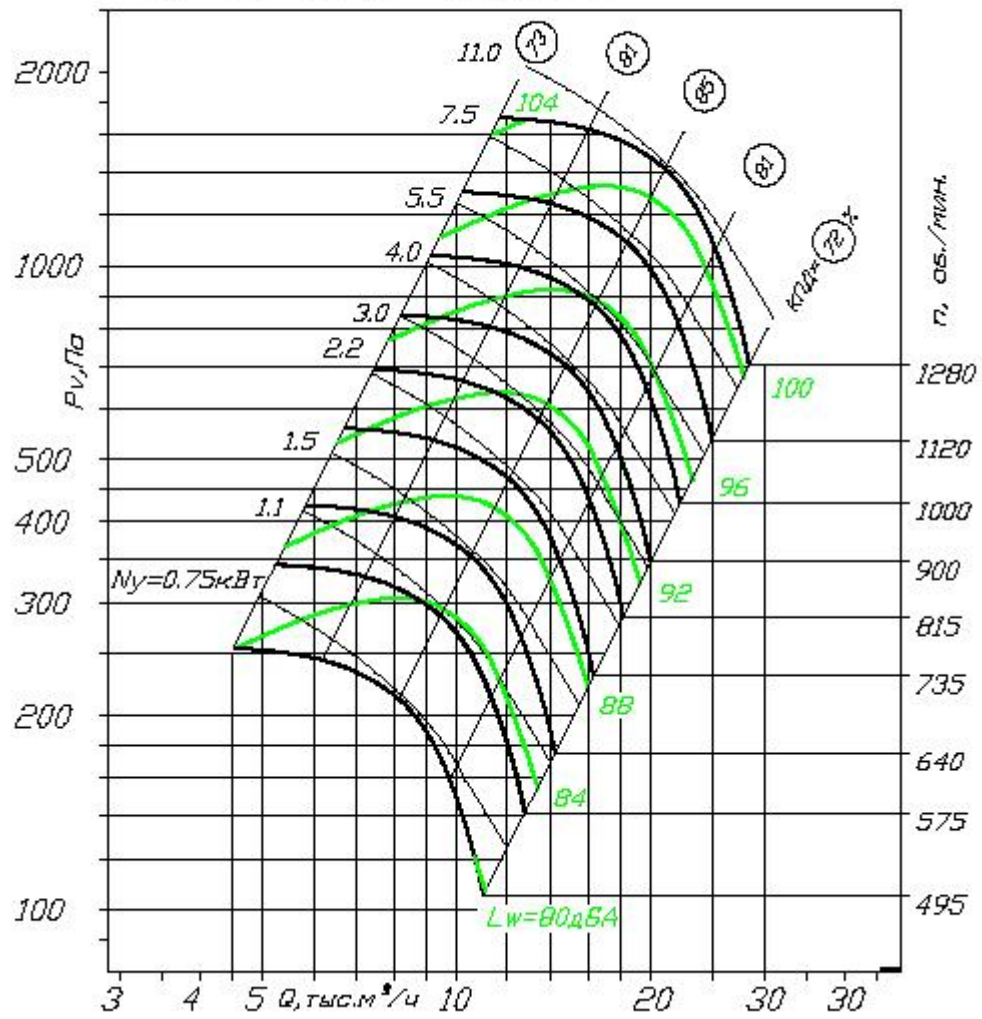
БР 80-75-8 схема 5
