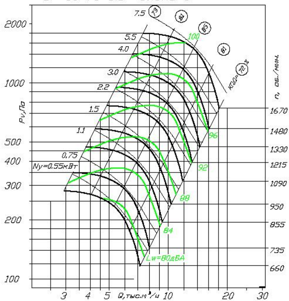
BP 80-75-6,3 схема 5
