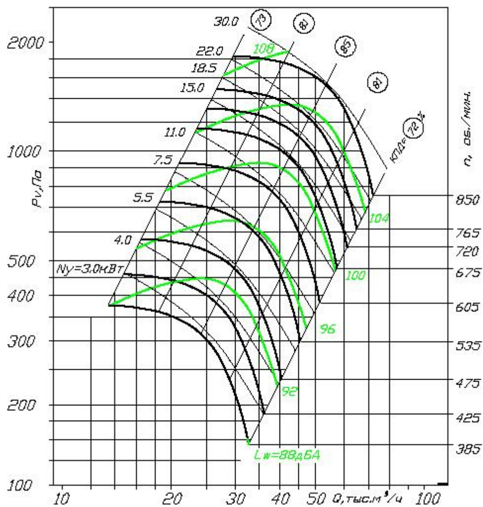
BP 80-75-12.5 схема 5
