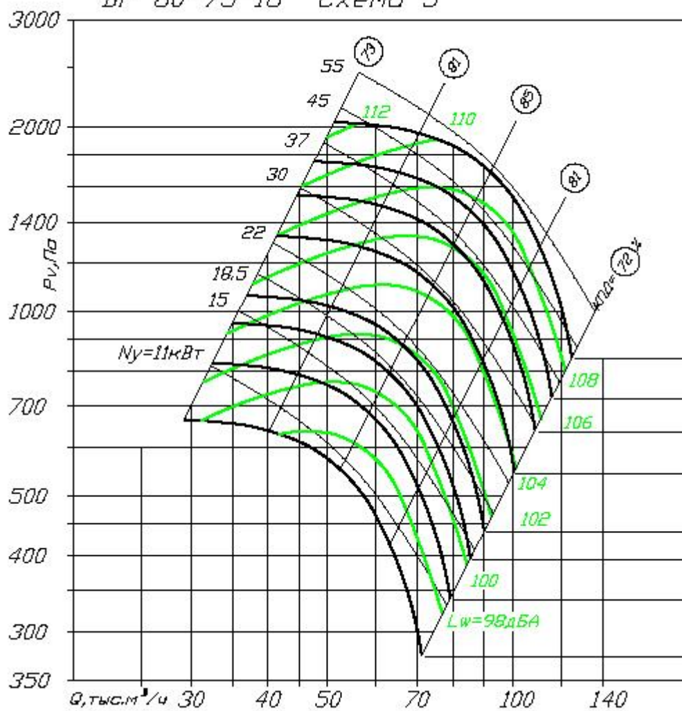
БР 80-75-16 схема 5
