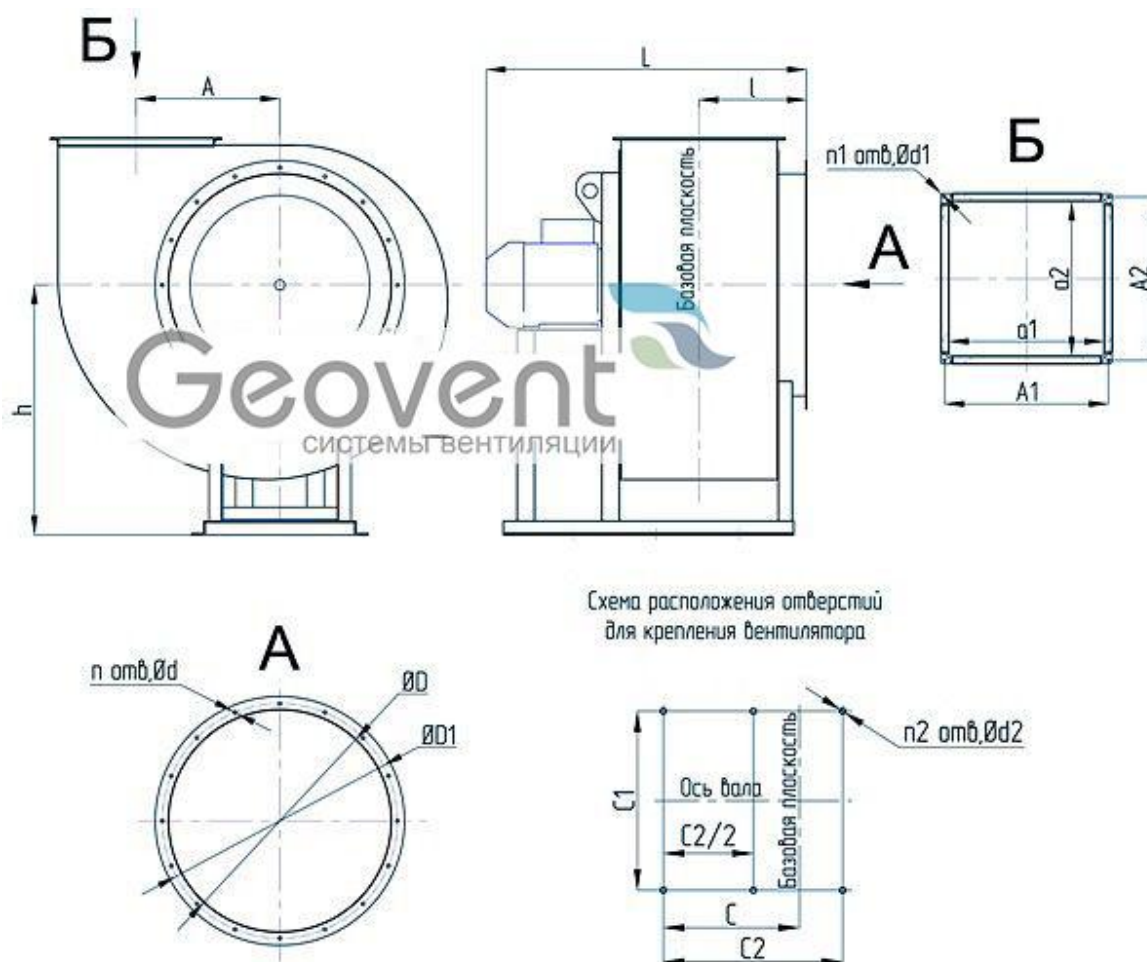
Габаритные и присоединительные размеры вентиляторов ВР 300-45 №2...8 исполнение 1
