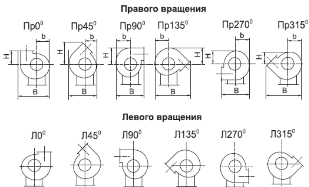
Положение кожуха вентилятора
