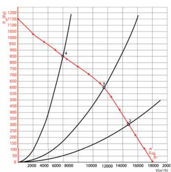
БКН 100-50/63-4D (380В)
