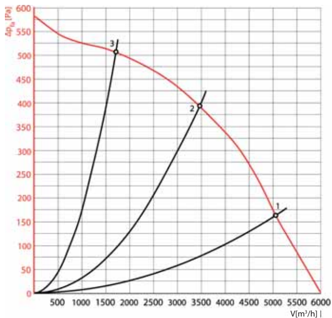
БКН 70-40/45-4D (380В)
