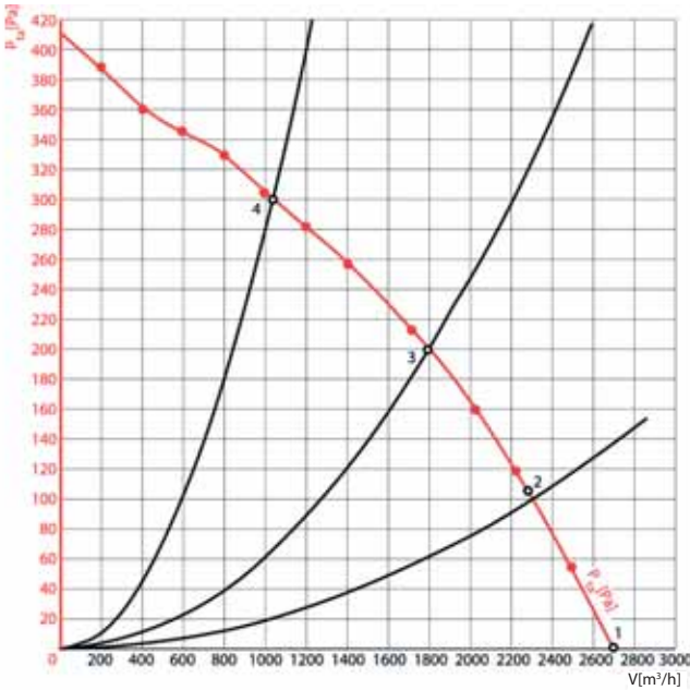
ВКН 60-30/35-4Е (220В)
