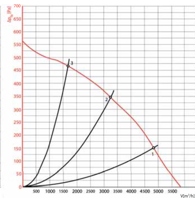
BKH 70-40/45-4E (220B)
