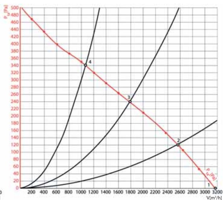
BKH 60-35/40-4E (220B)
