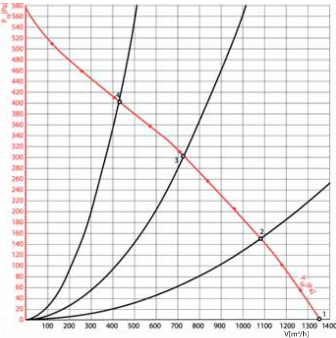
ВКН 50-25/25-2Е (220В)
